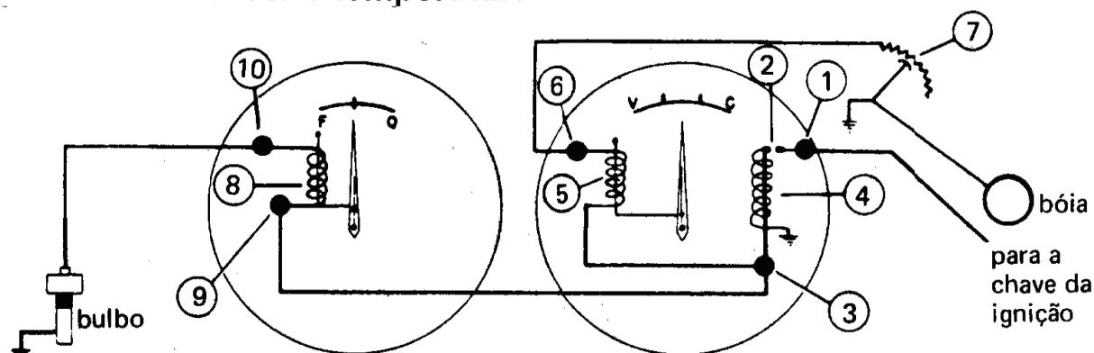
fig. 3 esquema dos indicadores de combustível e temperatura
